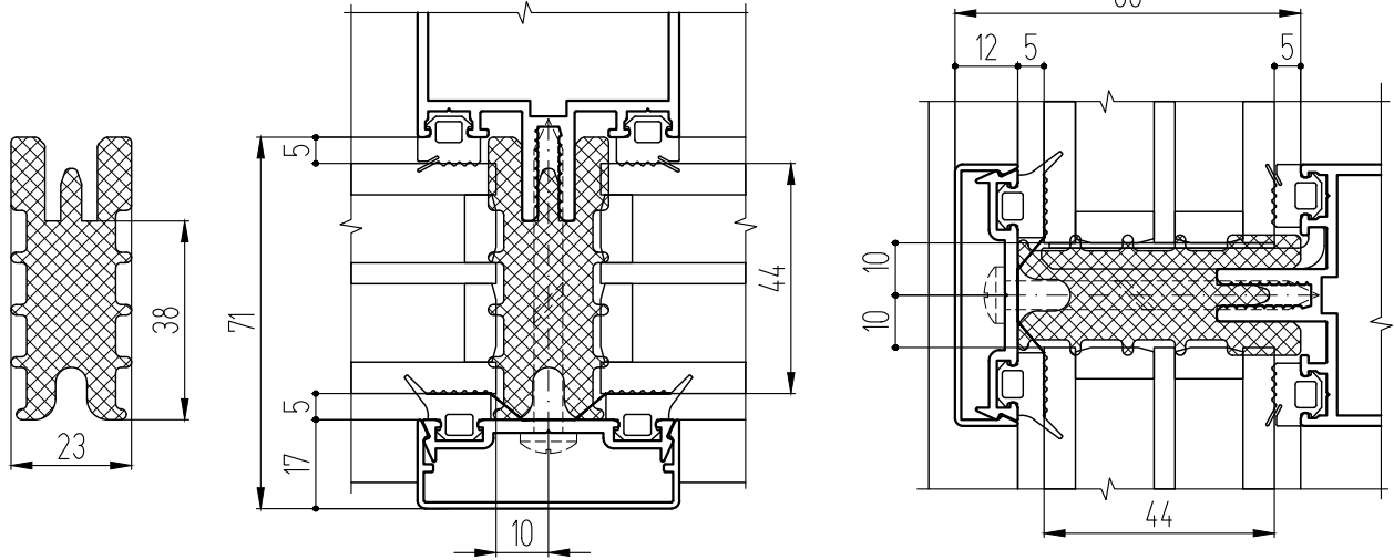
Заполнение 46 мм
