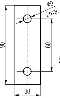
Шайба А45319-02
