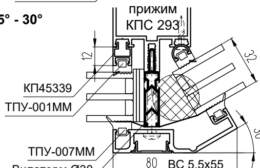
Для углов 30° - 37,5°
