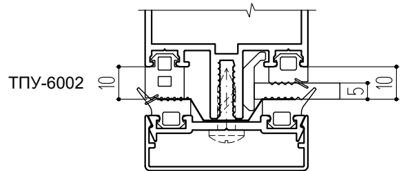
Заполнение 6 мм
