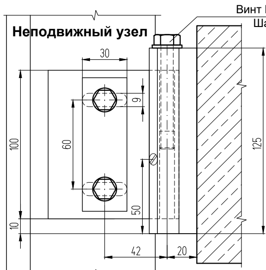
Шайба А45319-04
