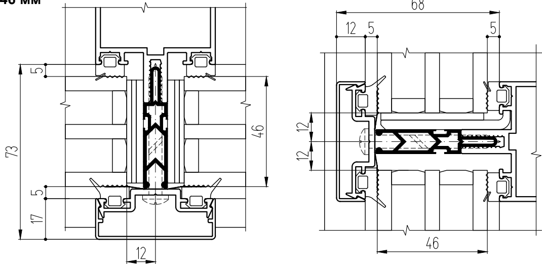
Заполнение 46 мм
