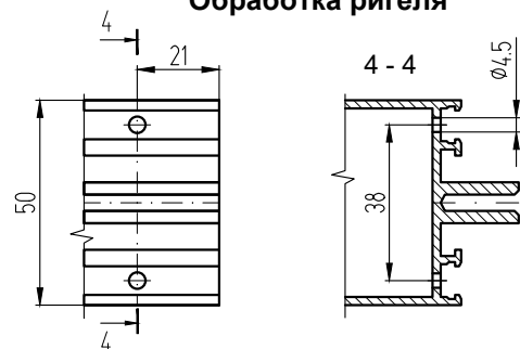
Обработка ригеля
