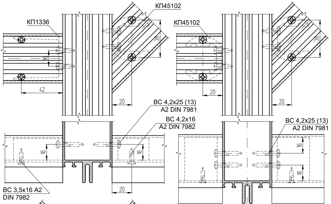
Обработка закладной КП45102
