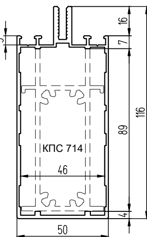
КП45551-3 (1,882 кг/м) J_x - 106,48, J_y - 26,26 W_x - 18,25, W_y - 10,5
