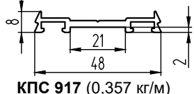
КПС 917 (0,357 кг/м)
