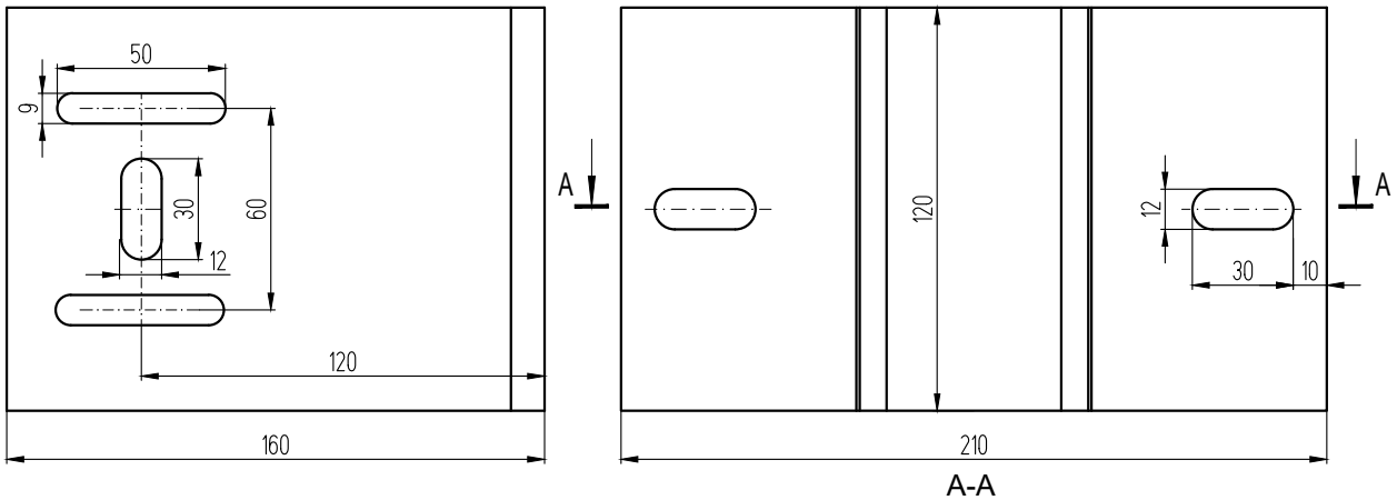
Шайба А268.01
