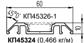
КП45324 (0,466 кг/м)
