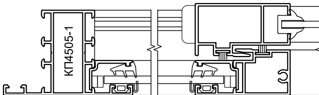
Однополосный слайдинг
