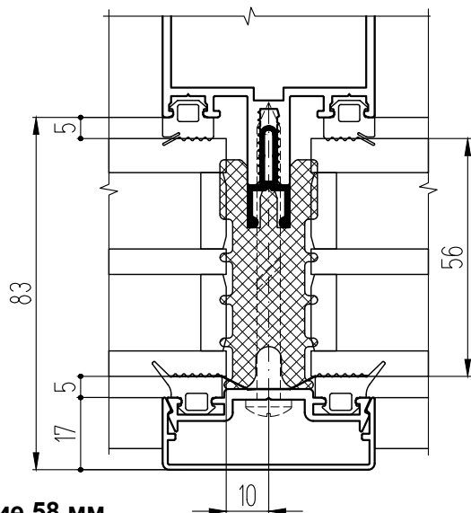
Заполнение 58 мм
