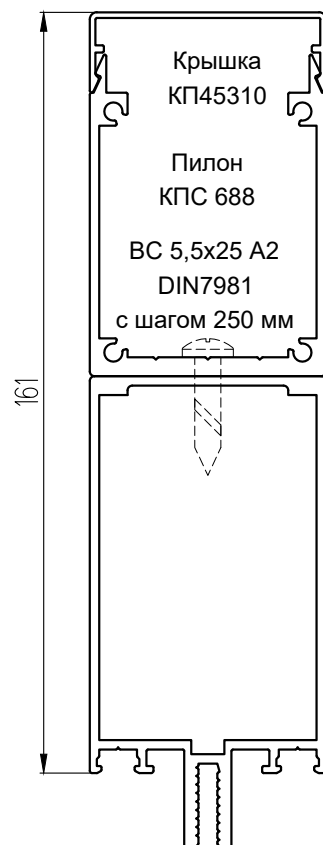
Усиление стоек витража при помощи внутреннего пилона КПС 688
