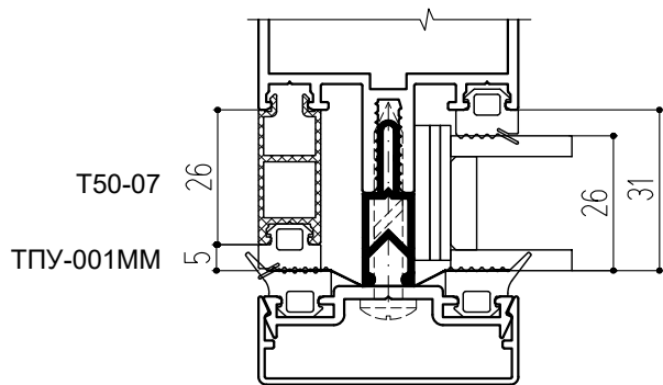
Заполнение 26 мм
