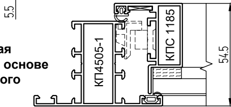
Структурная створка на основе ленты 3М
