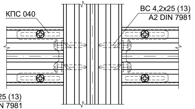
С закладной КПС 040
