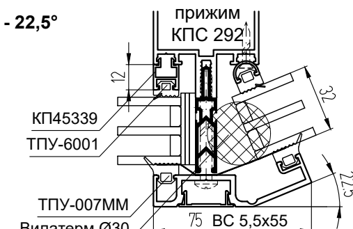
Для углов 22,5° - 30°
