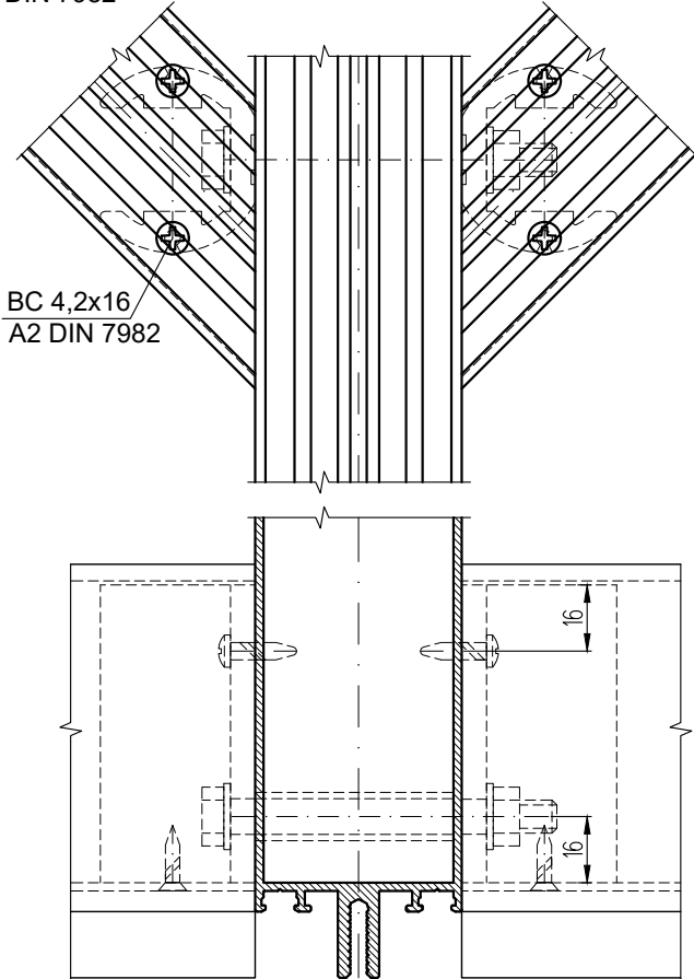
Обработка ригеля для угла 45° (крепление к закладной КП45102)
