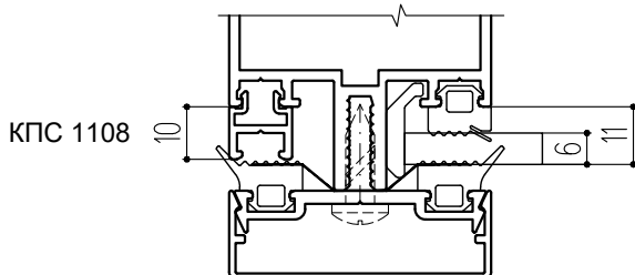
Заполнение 8 мм
