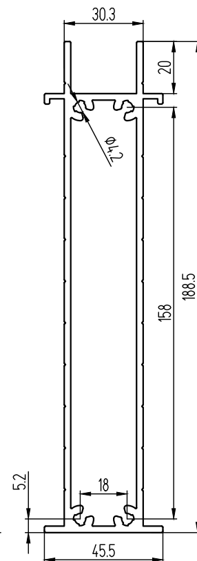
КПС 1069 (3,447 кг/м)
