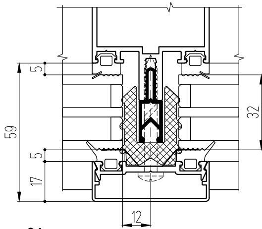
Заполнение 34 мм
