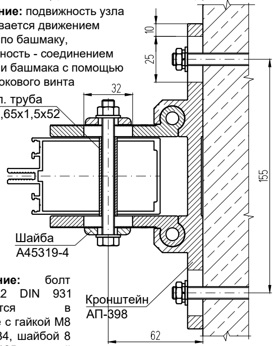
Обкладка КП45318 Для подвижных узлов
