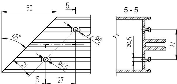
Обработка ригеля для угла 45° (крепление к закладной КП45102)
