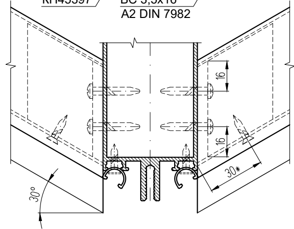
Обработка закладной КПС 040
