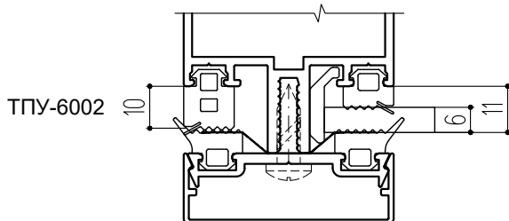
Заполнение 6 мм
