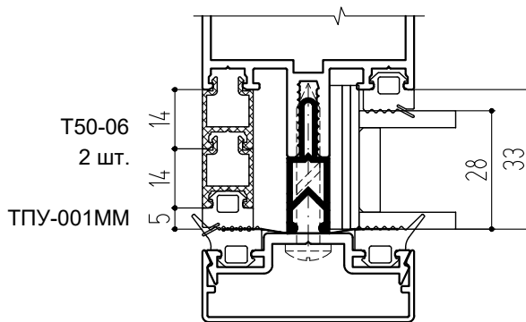
Заполнение 28 мм
