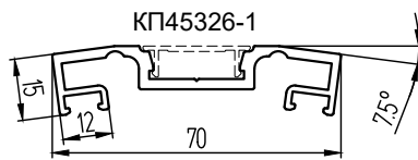
КПС 694 (0,82 кг/м)
