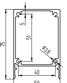
КПС 693-1 (1,361 кг/м)
