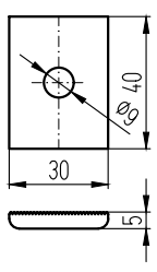
Шайба А45319-04
