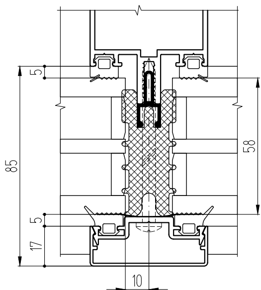
Заполнение 58 мм
